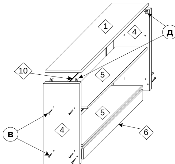
1 Схема сборки каркаса
