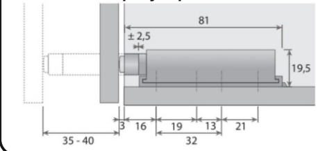
Установка и регулировка толкателя.
