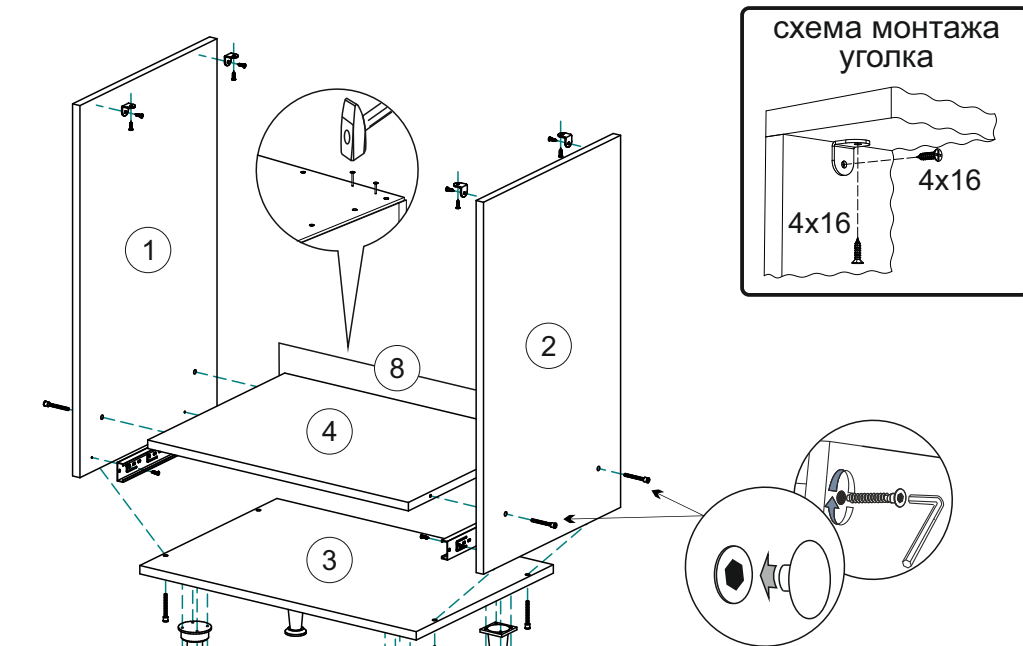
монтаж евроинта
